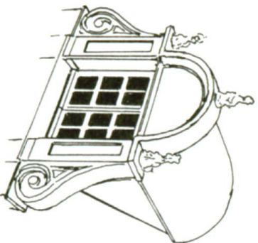
lucarne-fronton , ici à allèges et toit bombé
